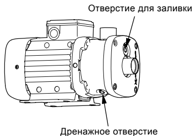
Рис. 8 Положение отверстия для заливки и дренажного отверстия
